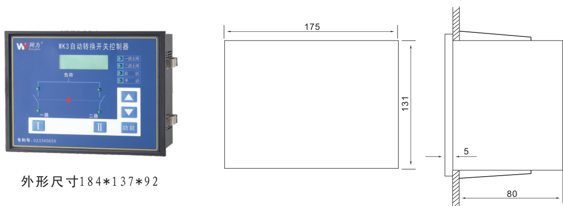
WK3网络型控制器安装开孔图
