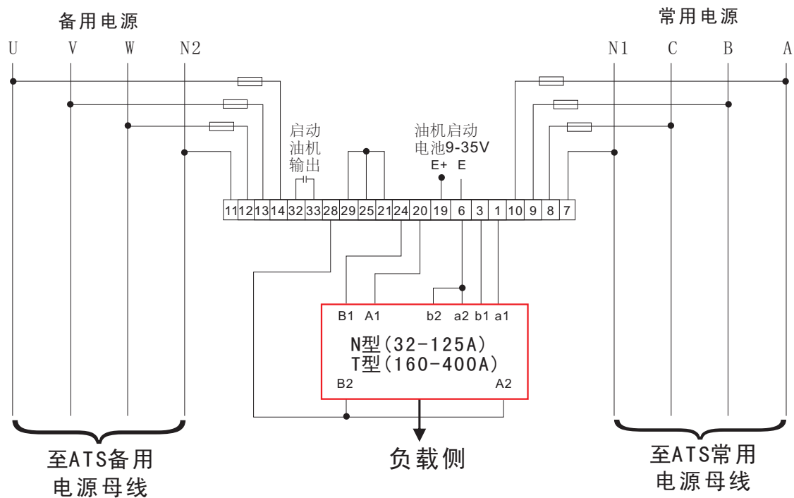
WK3网络型控制器与N型、T型ATS接线图
