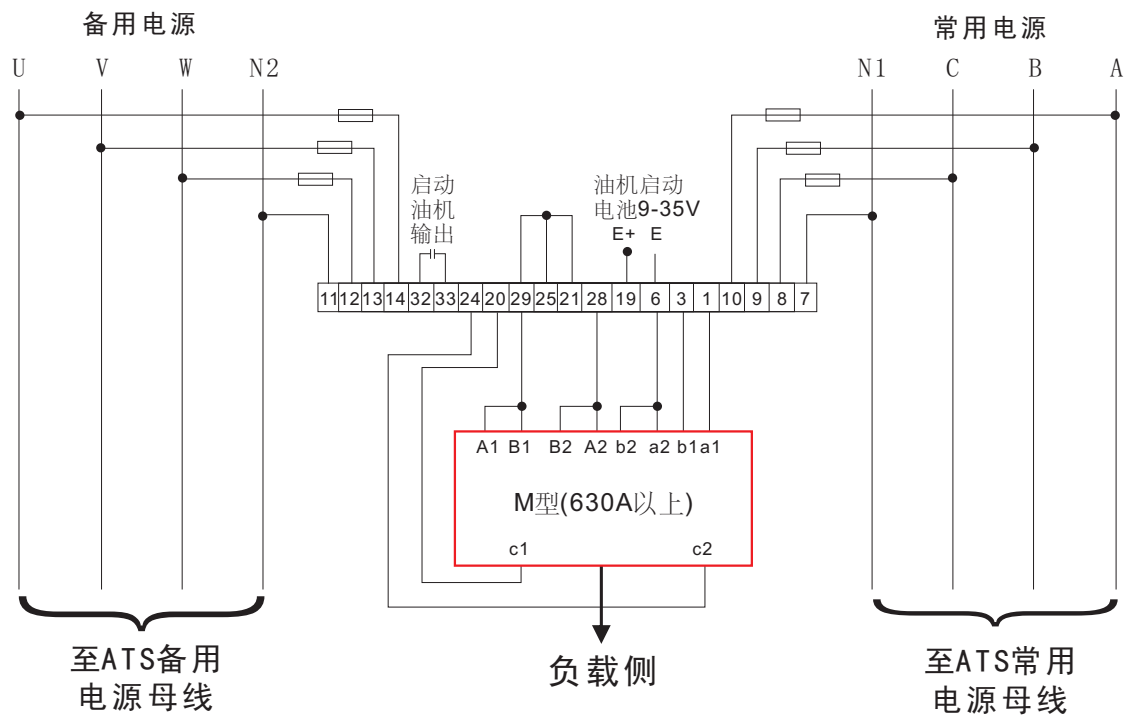
WK3网络型控制器与M型ATS接线图
