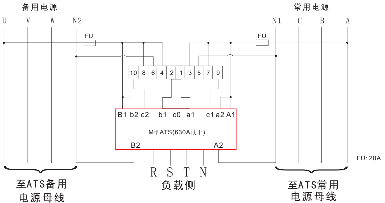
WK1终端型控制器与M型ATS接线图
