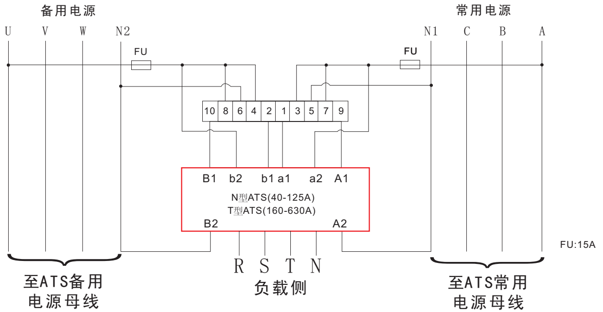
WK1终端型控制器与N型、T型ATS接线图
