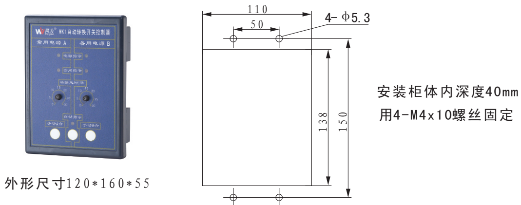
WK1终端型控制器安装开孔图
